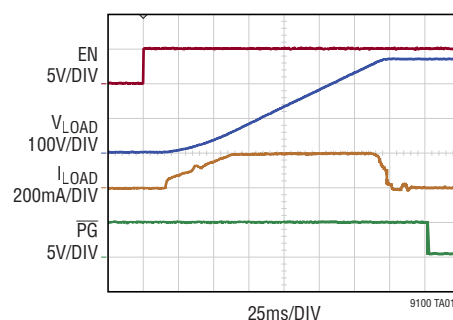
270V Load Soft-Start
